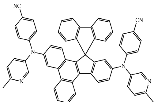
&lt;Compound 18A&gt;
