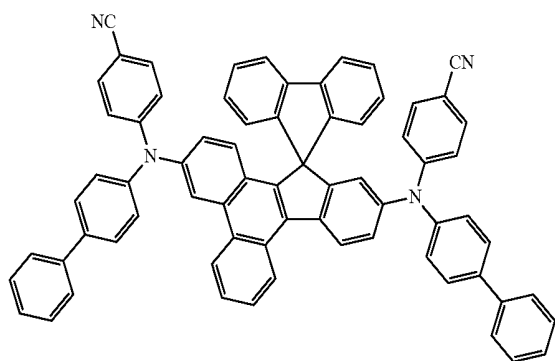
&lt;Compound 20A&gt;
