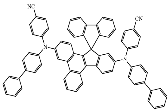
&lt;Compound 20A&gt;
